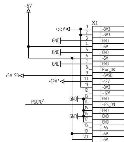
Разъем АТХ-питания
